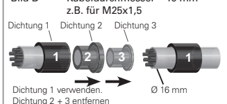
Bild D Kabeldurchmesser 16 mm
