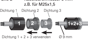
Bild B Kabeldurchmesser 9 mm
