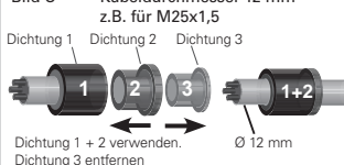
Bild C Kabeldurchmesser 12 mm
